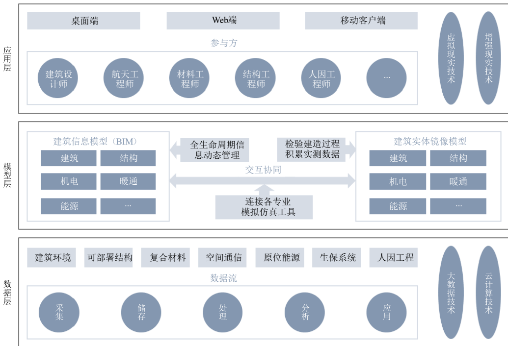
图 5 驻人月球科研站建筑设计系统工程的应用框架
