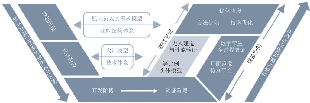
图7 驻人月球科研站建筑设计流程V字模型
