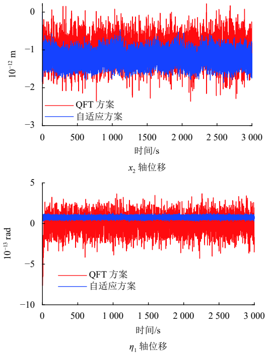
图4 与QFT方案的位移响应效果对比
