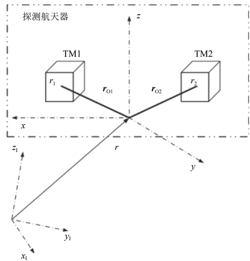
图1 LISA Pathfinder航天器多体动力学模型 [18]
