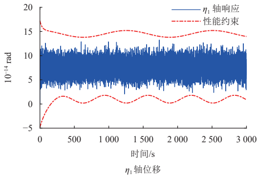
图5 性能约束的验证
