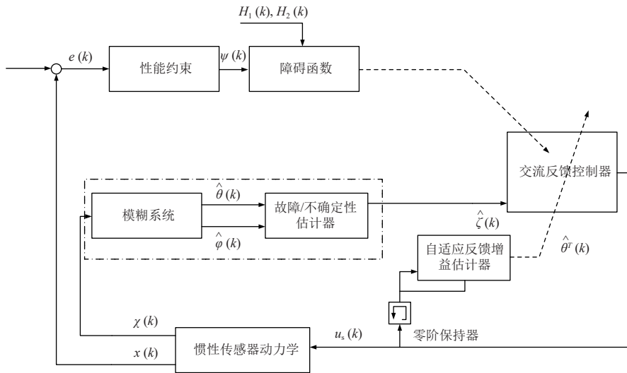
图2 控制结构 Fig. 2 Control framework
