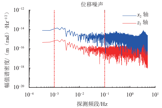
图3 非敏感轴频域位移响应
