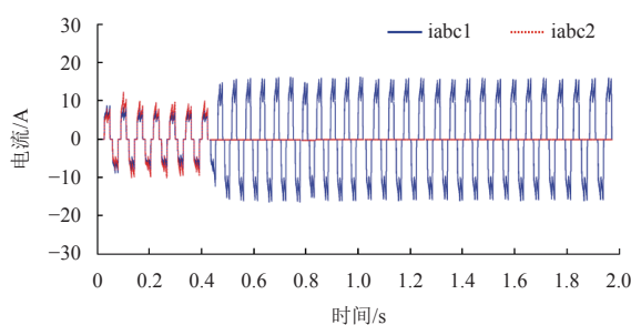
(b) 主份与备份A相绕组电流仿真波形
