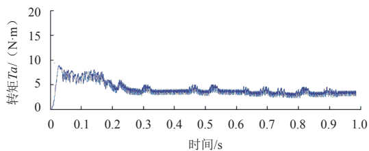
(d) T_a 输出转矩
