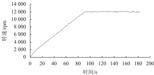
图 17 电机速度曲线 Fig. 17 Motor speed
