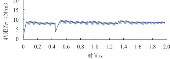
(e) T_e 输出转矩
