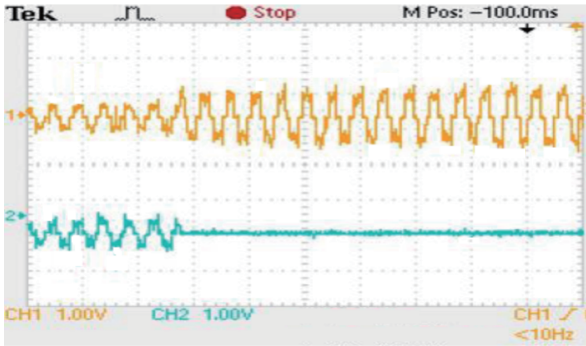
图 18 绕组电流波形曲线 Fig. 18 Winding current
