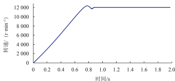
(a) 转速仿真波形
