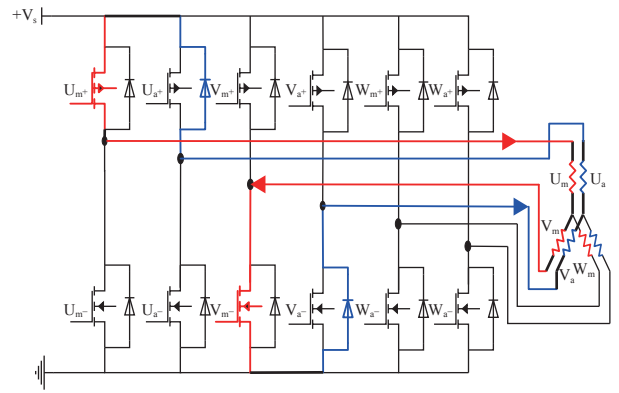
图5 两相绕组驱动电路耦合工作电流回路
