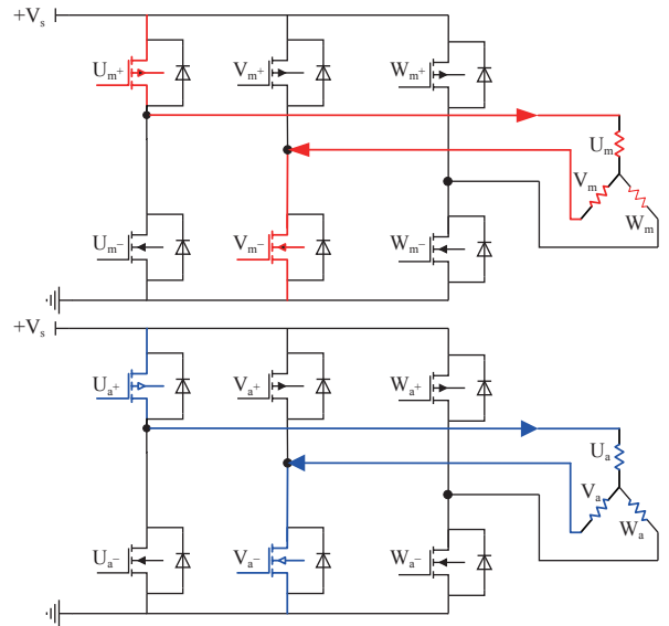
图6 两相绕组驱动电路独立工作电流回路
