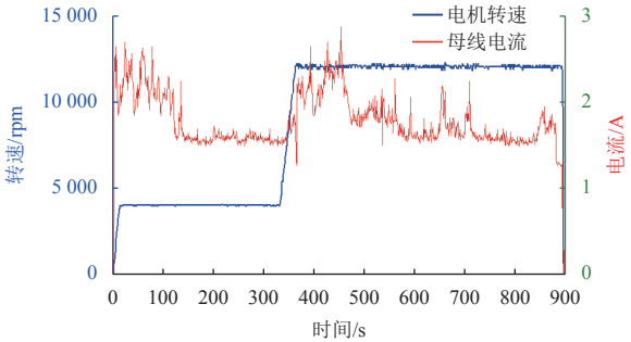
图 20 转速和母线电流关系曲线 Fig. 20 Spinning speed and bus current
