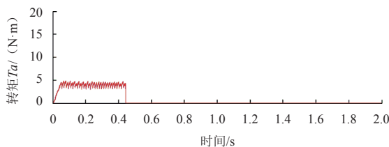
(d) T_a 输出转矩
