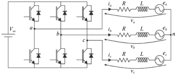
图4 三相直流无刷电机等效电路
