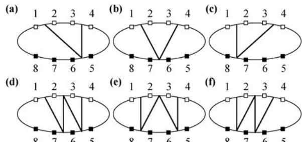
Fig. 7 Six zigzag diagrams for A_8(1^-, 2^-, 3^-, 4^-, 5^+, 6^+, 7^+, 8^+) .
