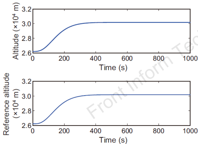
Fig. 4 Altitude tracking
