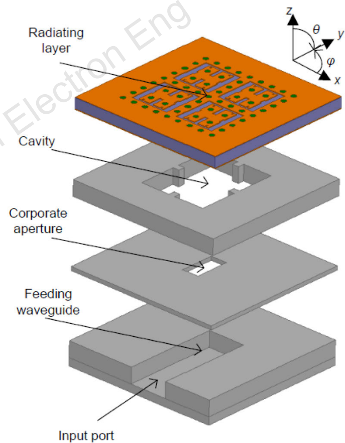
Fig. 17 Configuration of the 2 \times 2 antenna subarray
