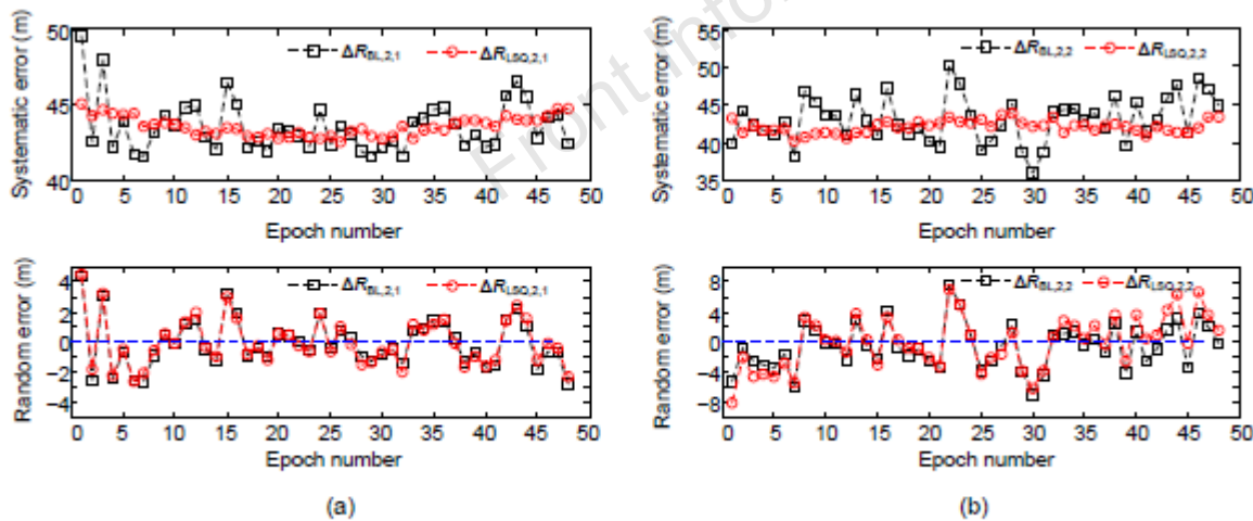
Fig. 8 Error calibration of B2: (a) \varepsilon_{BL,2,1}=1.5 ; (b) \varepsilon_{BL,2,1}=3
