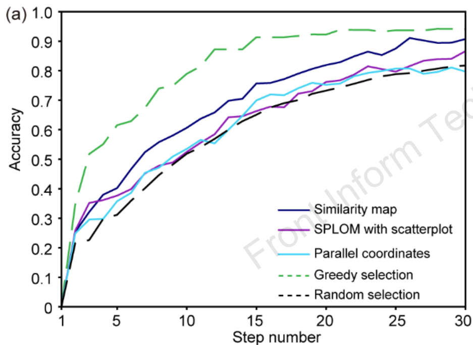
MNIST4
