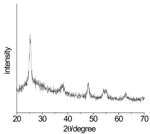
Fig. S1 XRD pattern of the TiO 2 nanowires
