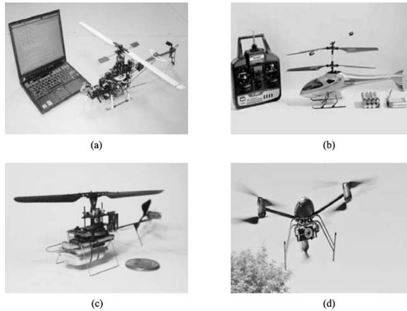
Fig. 7 Type III RC rotorcraft. (a) Trex-450; (b) Lama-V4; (c) PD-100 Black Hornet; (d) Draganflyer
