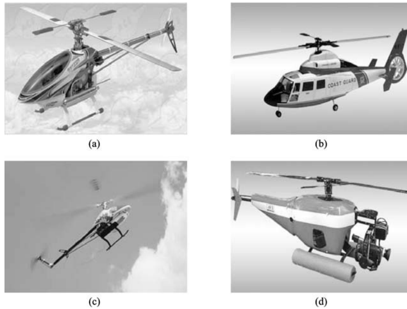
Fig. 6 Type II RC rotorcraft. (a) Raptor 90 SE; (b) Dauphin; (c) Maxi-Joker 2; (d) Observer-Twin
