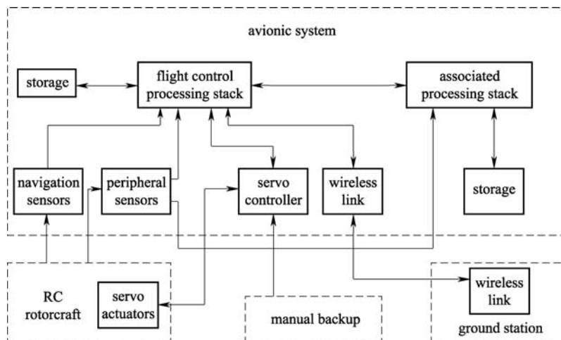
Fig. 2 System configuration of a mini rotorcraft UAV
